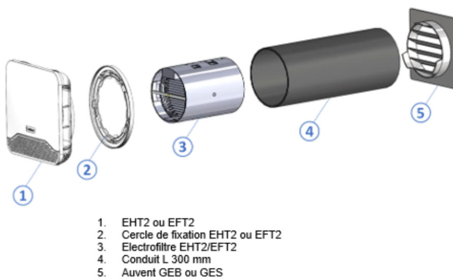
Figure 22a – Mise en œuvre des entrées d'air EHT2 ou EFT2 avec électrofiltre EHT²/EFT² sans mousse Ø 125 mm L 300 mm
