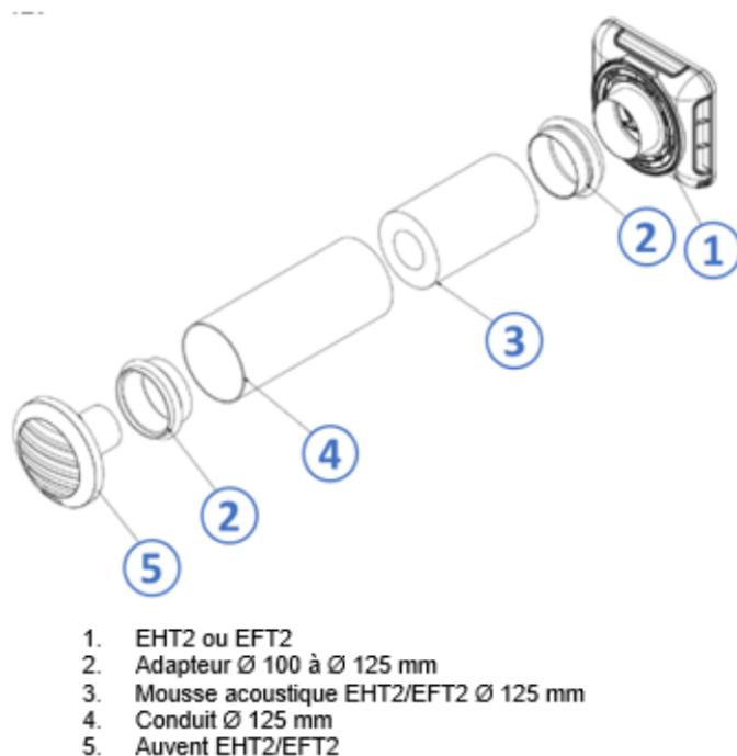
Figure 21c – Mise en œuvre des entrées d'air EHT² ou EFT² en conduit Ø 125 mm L 300 mm
